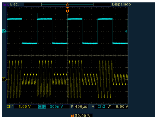
Figura 6. Señales (A=0.5V)
